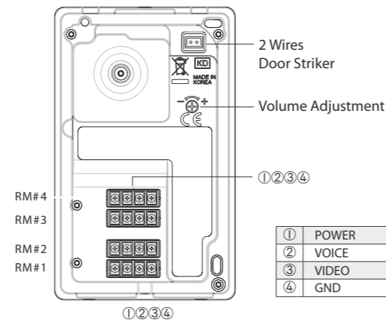
* WIRING (EX. UDP-604/614)
