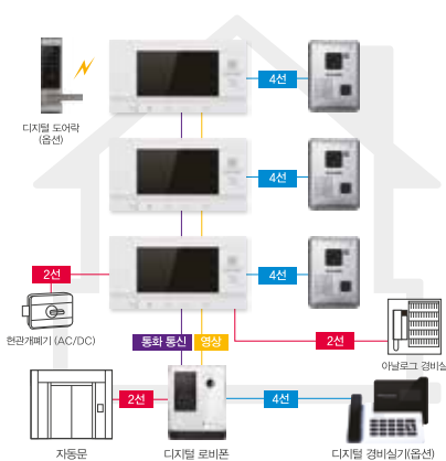
단독주택/아파트 설치구성도
